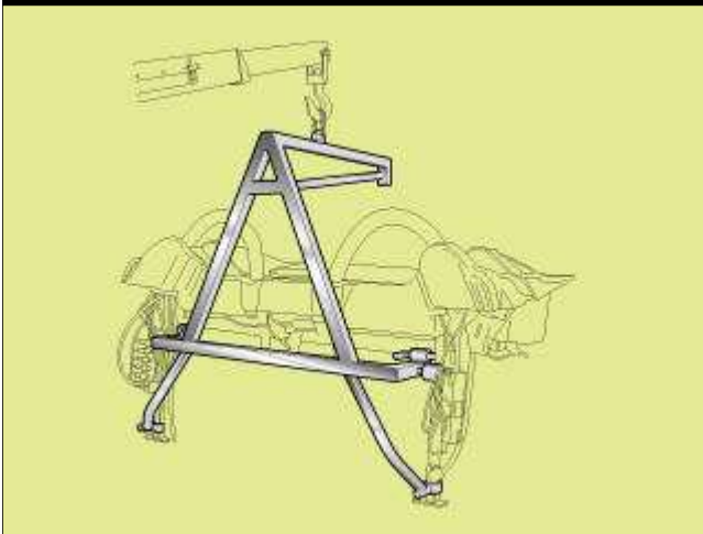
● 框架 95975736 (AV 5736) 用于升起硬顶。
